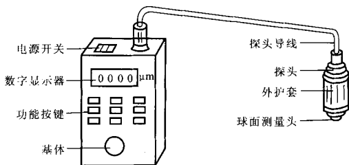
图1 数字式电涡流测厚仪
