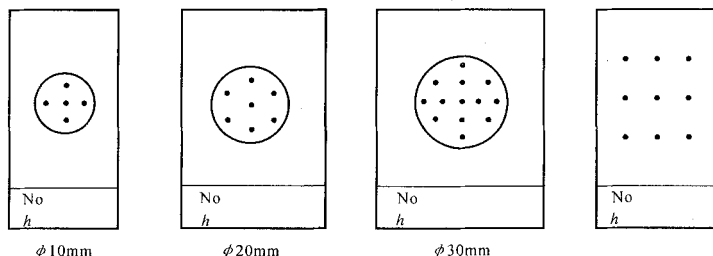
图 3 校准用厚度片受检区域及受检点数示意图
