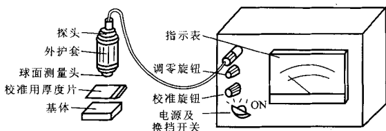
图2 指示表式电涡流测厚仪
